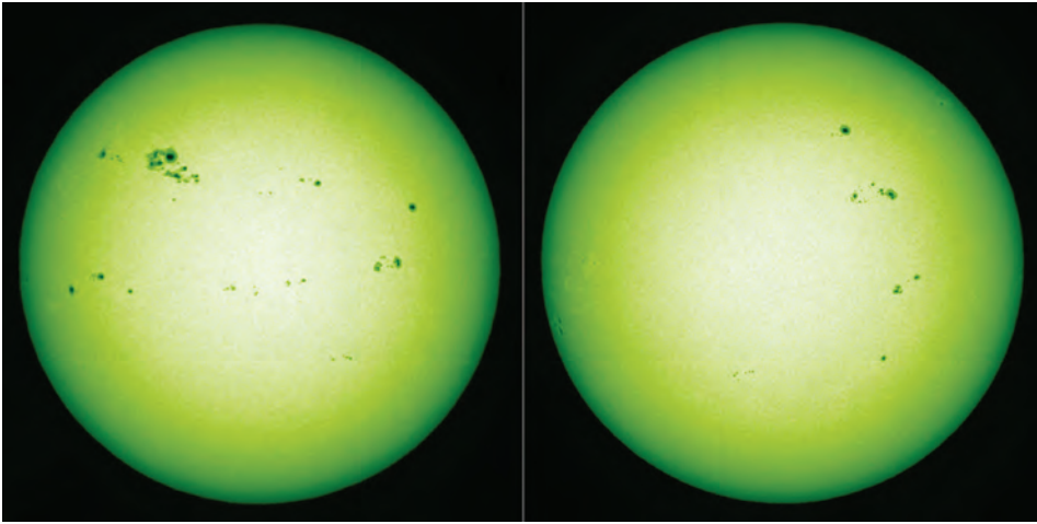
2001年3月(左)と12年10月に撮影された太陽の様子。左は前の周期で最も黒点数が多かった時期(国立天文台太陽観測所提供)
