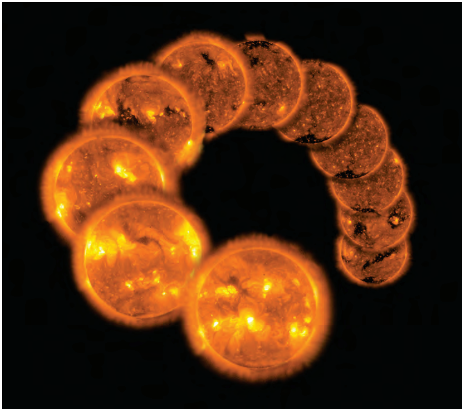
太陽観測衛星「ひので」が、2007年4月（右奥）から12年4月（手前）にかけて半年ごとに捉えた太陽の画像。10年ごろから活動は高まりつつあるが、通常よりも低調（国立天文台・JAXA提供）
