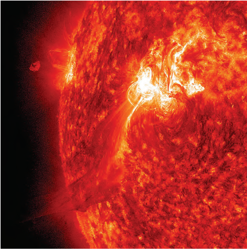
2011年9月に米太陽観測衛星「SDO」が撮影した太陽表面の爆発(フレア)(NASA提供)
